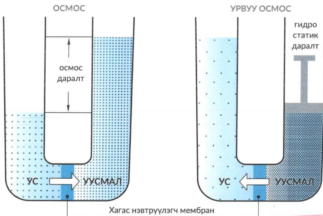
Зураг 7. Урвуу осмосын үйл явц
