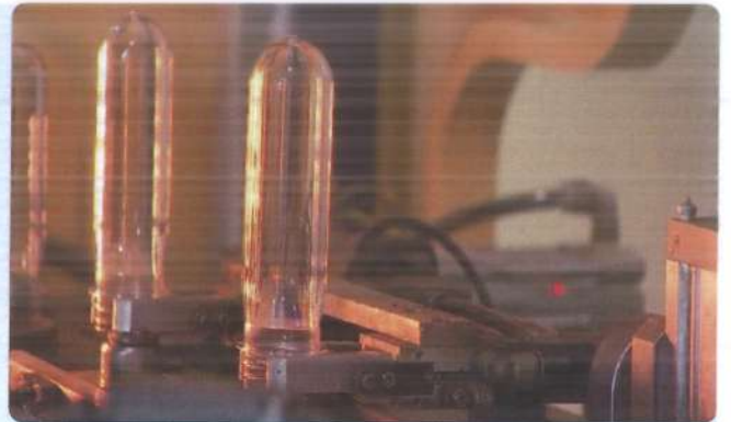
Хуруу савыг үлээх төхөөрөмж рүү оруулах
