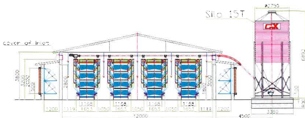
Зураг 18 Өндөглөгчийн байрны план зураг
