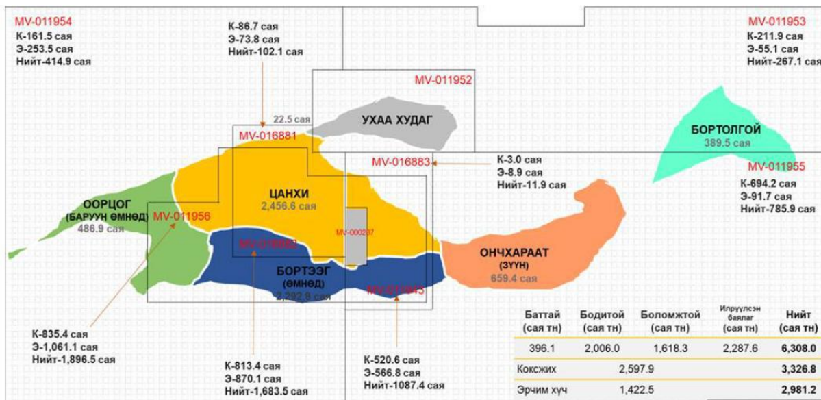
Зураг 2. Тавантолгой бүлэг ордын ордуудын байршил, тусгай зөвшөөрөл
