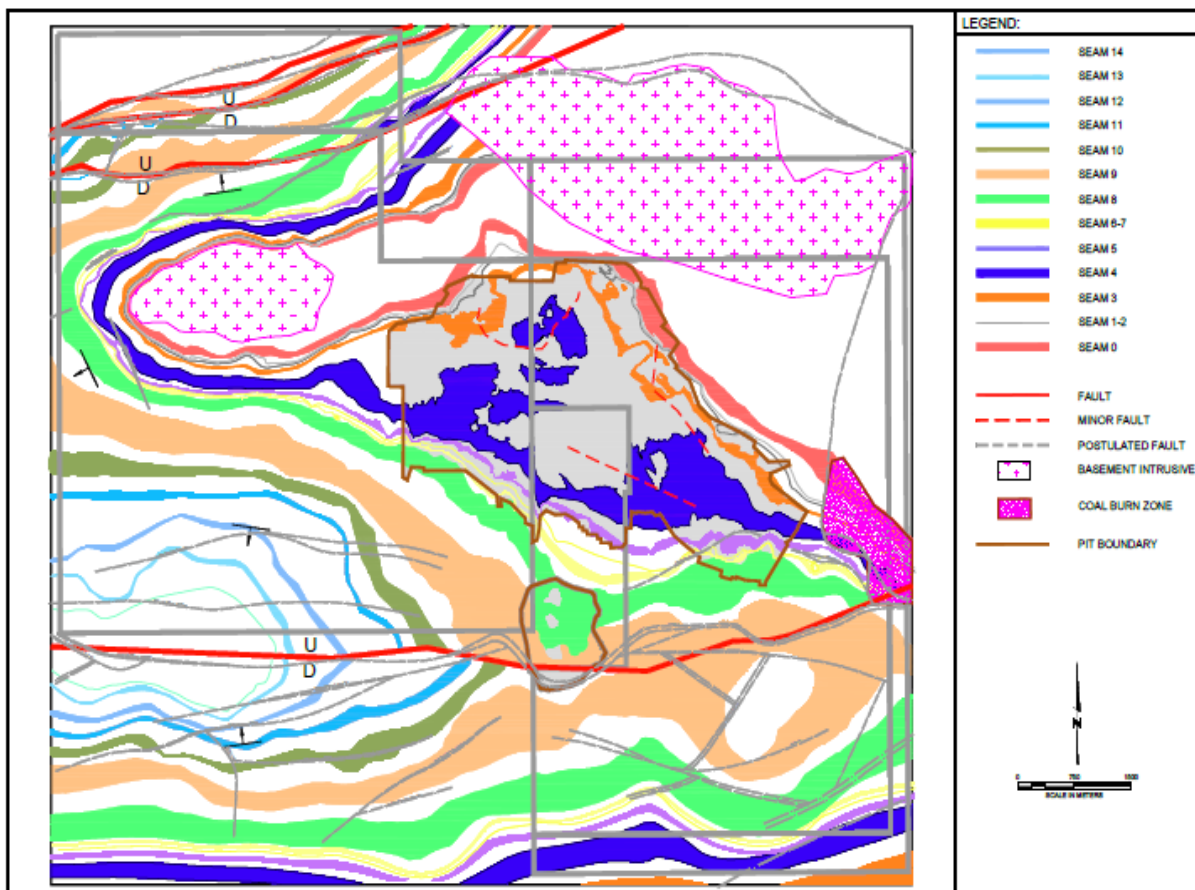
Зураг 3. Цанхийн хэсгийн нүүрсний давхраасуудын тогтоц
