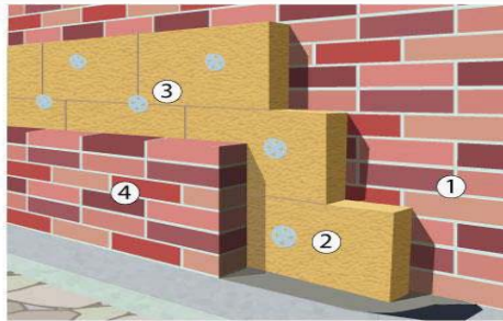
1. Бетонон хана (тоосго пено бетон) 2. Basaltwool чулуун хөвөн хавтан, 3. Шаантан тогтоогч, 4. Гадна өнгөлгөөний тоосгон хана
