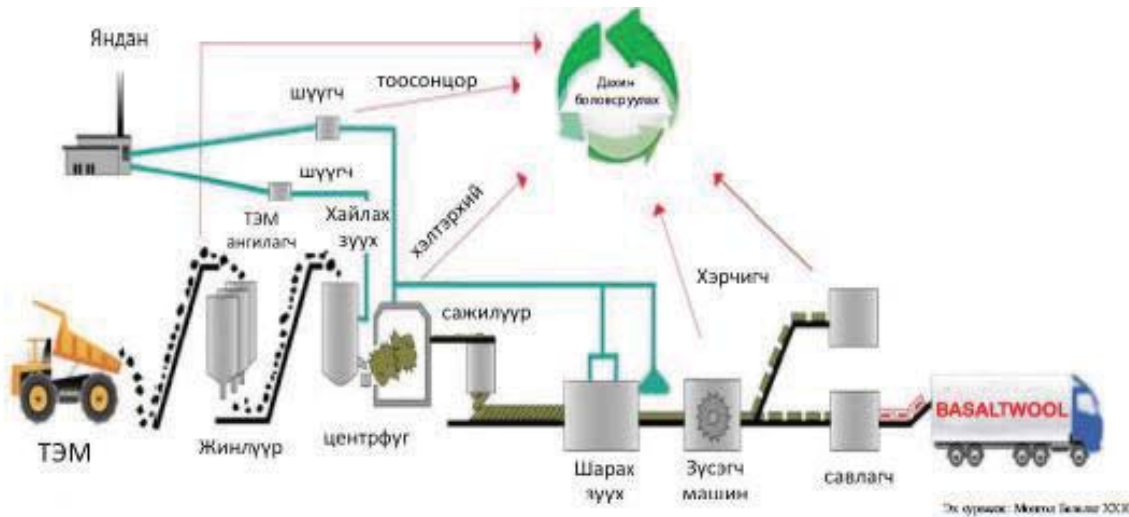
Зураг 15 Үйлдвэрийн схем
