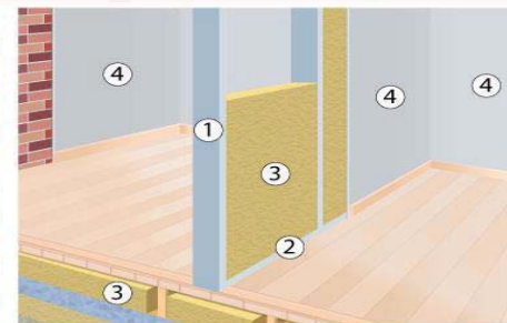
1. С төмөр багана, 2. С төмөр чиглүүлэгч, 3. Basaltwool чулуун хөвөн хавтан, 4. Гипсэн хавтан
