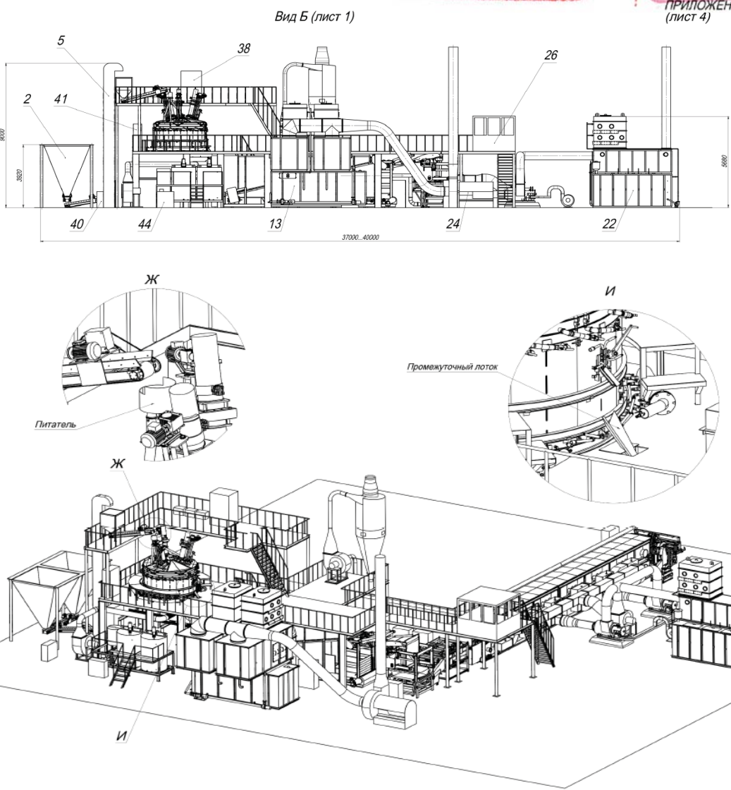
Зураг 51 Үйлдвэрийн шинэчлэлийн бүдүүвч зураг
